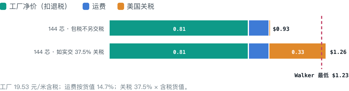
图 8 144 芯落地成本拆解（美元/英尺）
